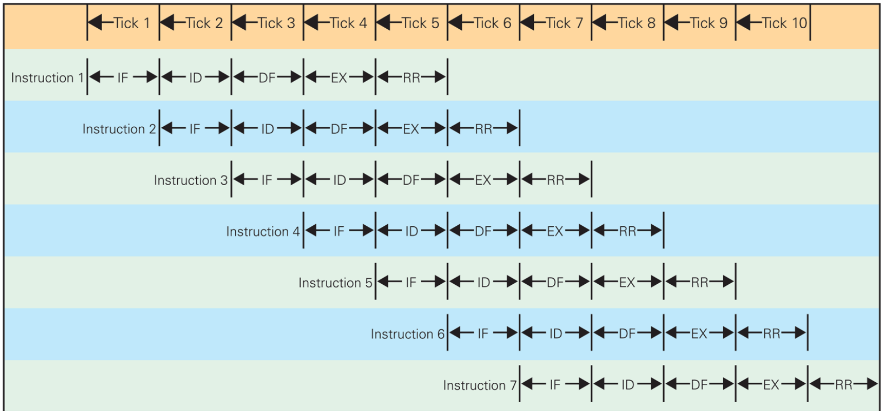
Figur 9.12 Skjematiske diagram for en parallell-prosessert «pipeline» Hente/Eksekvere «F/E»-syklus. På hvert tikk starter IF en ny instruksjon, og sender den deretter videre til ID (Instruksjons-Dekoding) enheten; ID-enheten arbeider med instruksjonen den fikk, og når den er ferdig sendes instruksjonen videre til DF (Datahenting «Fetch»)-kretsen, og så videre. Mens «røret» er fullt utføres fem instruksjoner samtidig, og en instruksjon blir ferdig på hvert klokke-tikk, som gjør at det ser ut som om maskinen kjører en instruksjon per tikk.
