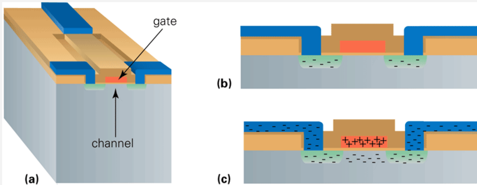
Figur 9.18 Virkemåten til en felt-effekt transistor. (a) Tverrsnitt av transistoren fra Figur 9.14f. (b) Porten (rød) er nøytral og kanalen (Silisiumregionen rett under porten) leder ikke strøm, men isolerer ledningene (blå); (c) Ved å «lade» porten begynner kanalen og lede, og ledningene blir dermed «sammenkoblet».
