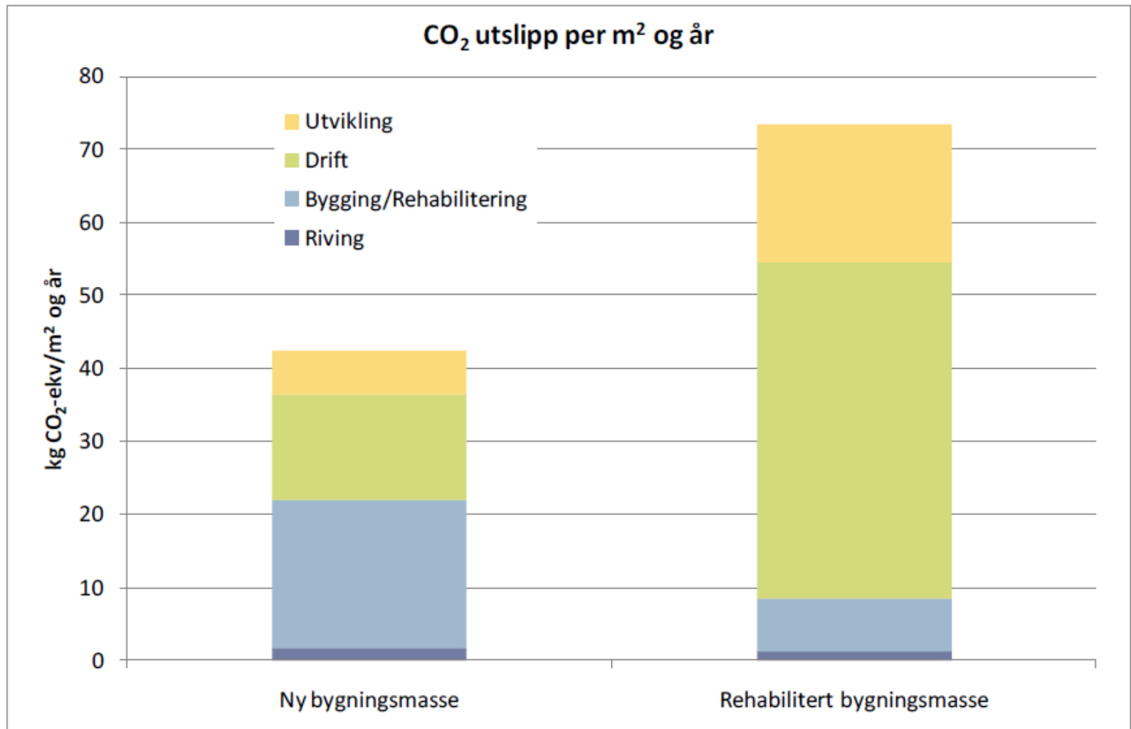
Figur 3.2 CO 2 -utslipp per m 2 og år for ny og rehabilitert bygningsmasse.
