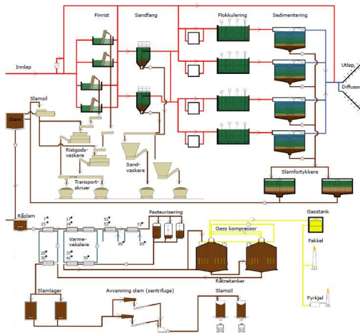
Flytskjema
